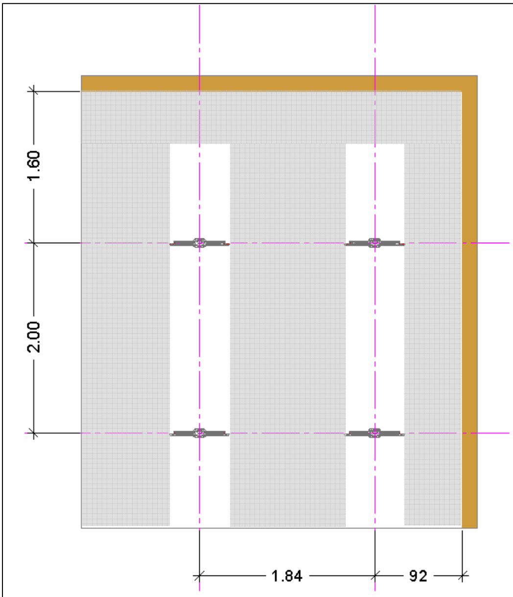
Abb.2: Mindestgeräteabstände im Raum
